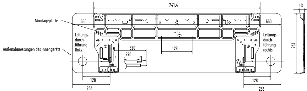
Frontansicht
