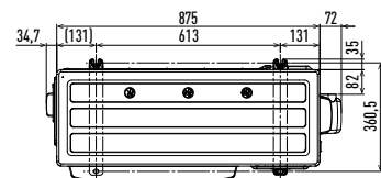
Frontansicht
