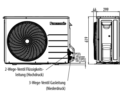
Frontansicht
