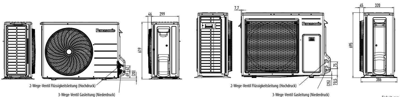
Seitenansicht
