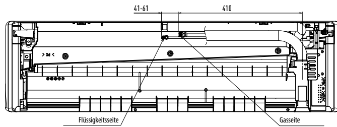
Anordnung von Innengerät und Montageplatte
