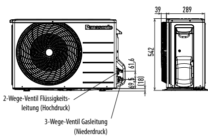
Frontansicht
