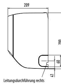
Seitenansicht
