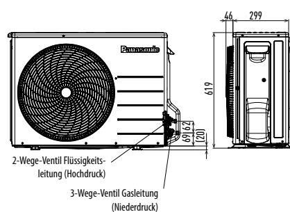
Frontansicht
