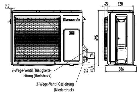
Frontansicht
