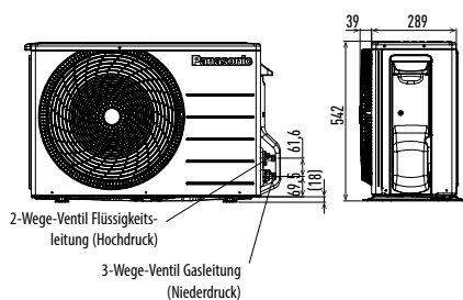
Frontansicht
