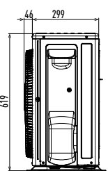
Seitenansicht
