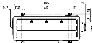
Draufsicht
