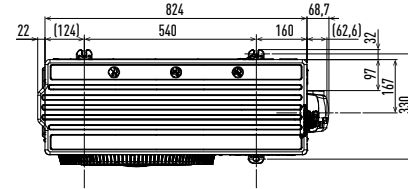
Frontansicht
