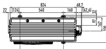
Frontansicht
