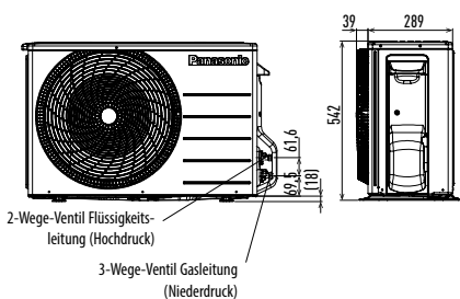
Frontansicht
