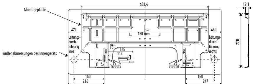
Anordnung von Innengerät und Montageplatte Frontansicht
