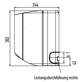
Seitenansicht
