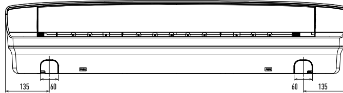
Rückansicht
